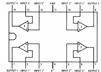
LM2902 (4x Op. Amp.)
