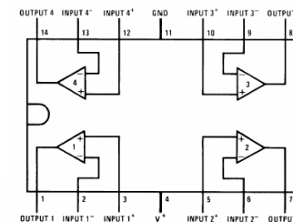
LM2902 (4x Op. Amp.)
